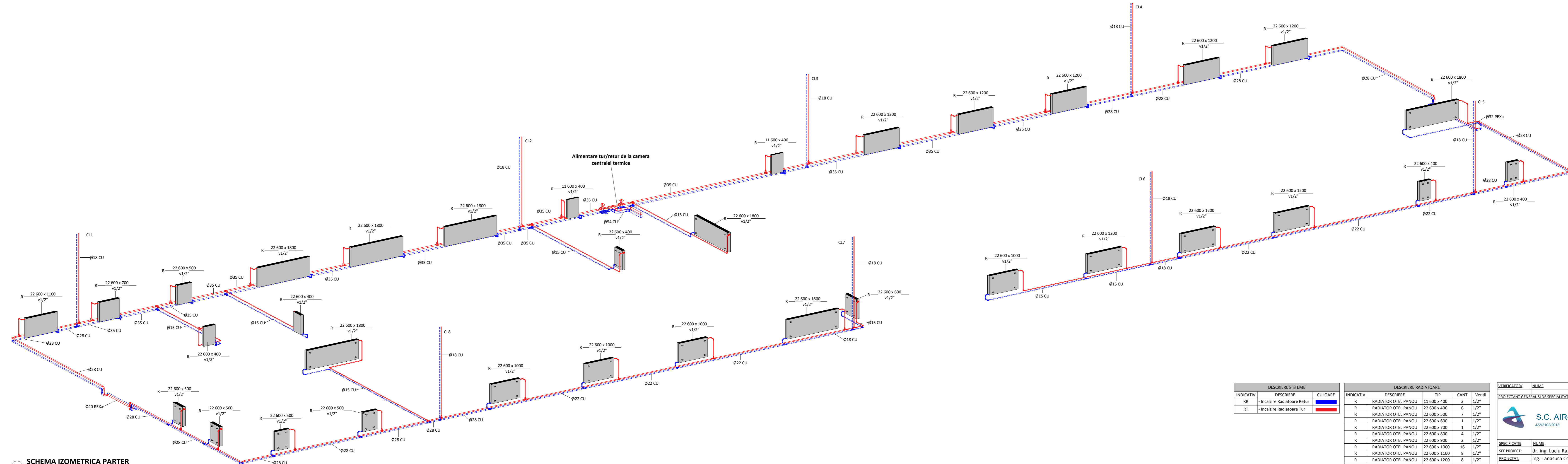
1 SCHEMA IZOMETRICA PARTER
