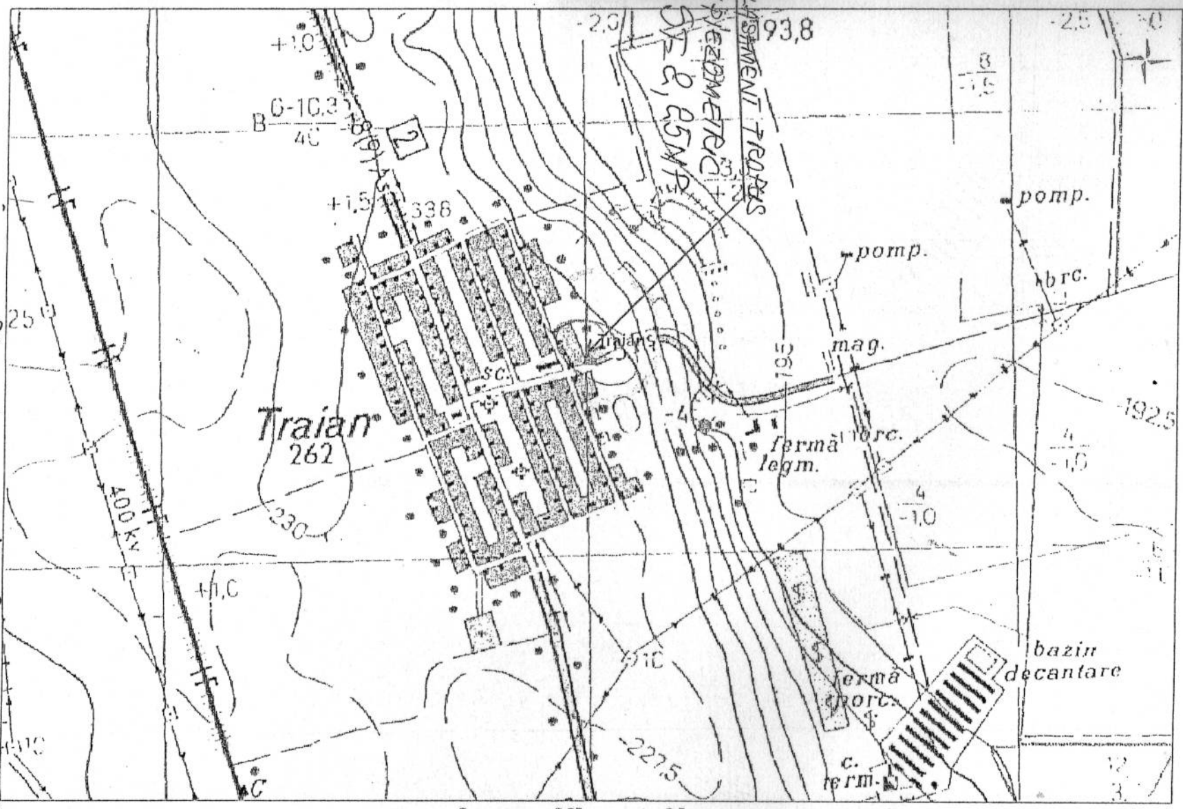
Plan de situatie cu incadrarea in zona a forajului Traian, jud. Neamt
